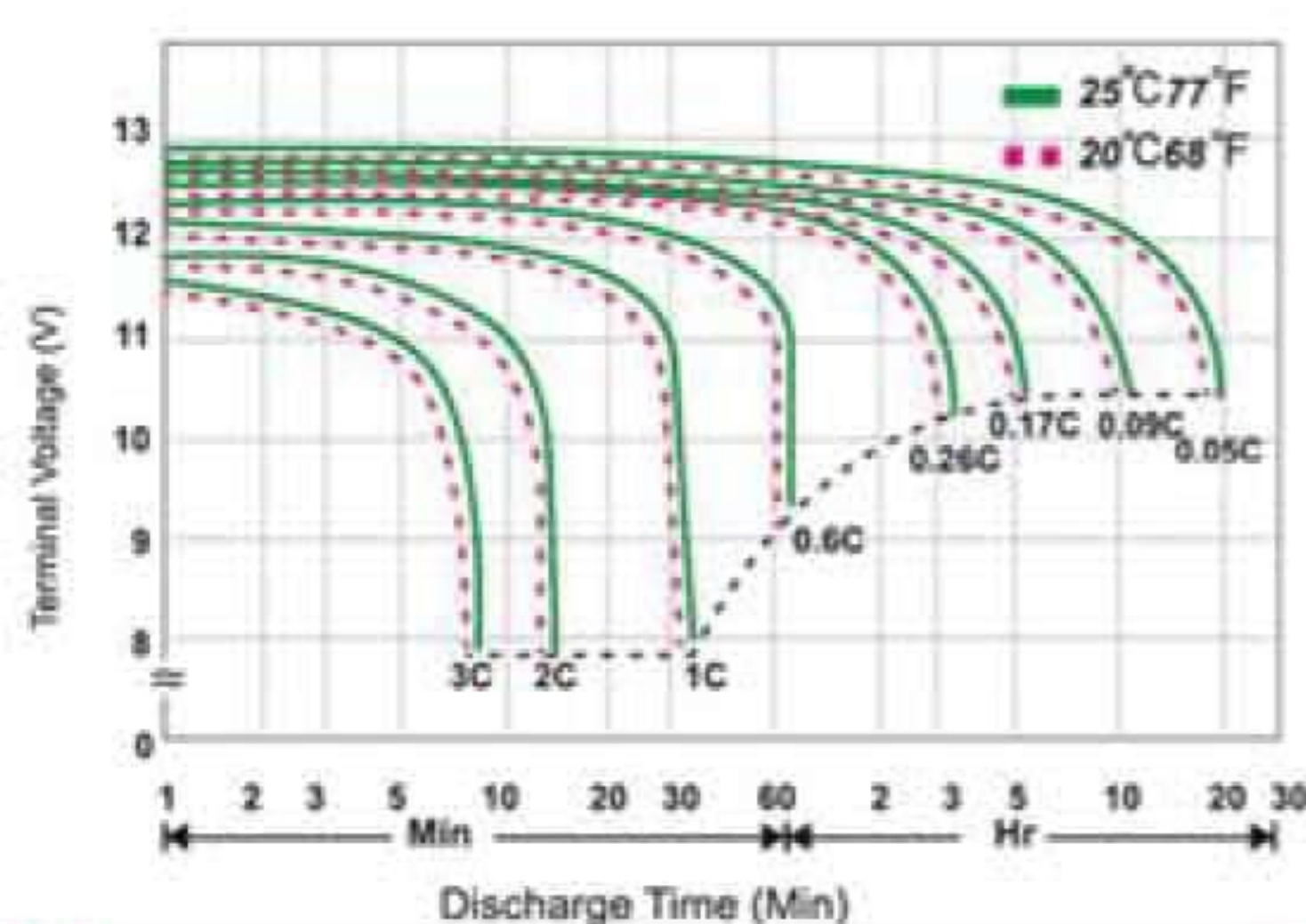
نمودار دشارژ
