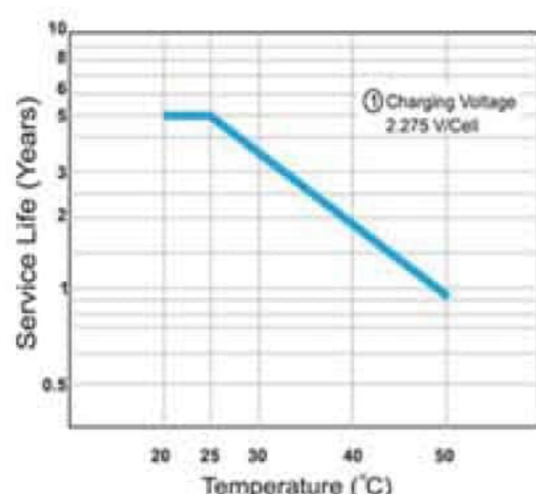
نمودار طول عمر در دمای متغیر
