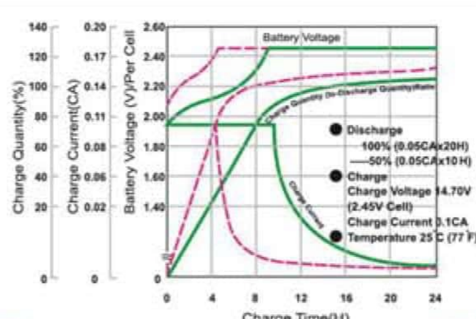
نمودار منحنی شارژ در حالت استفاده
