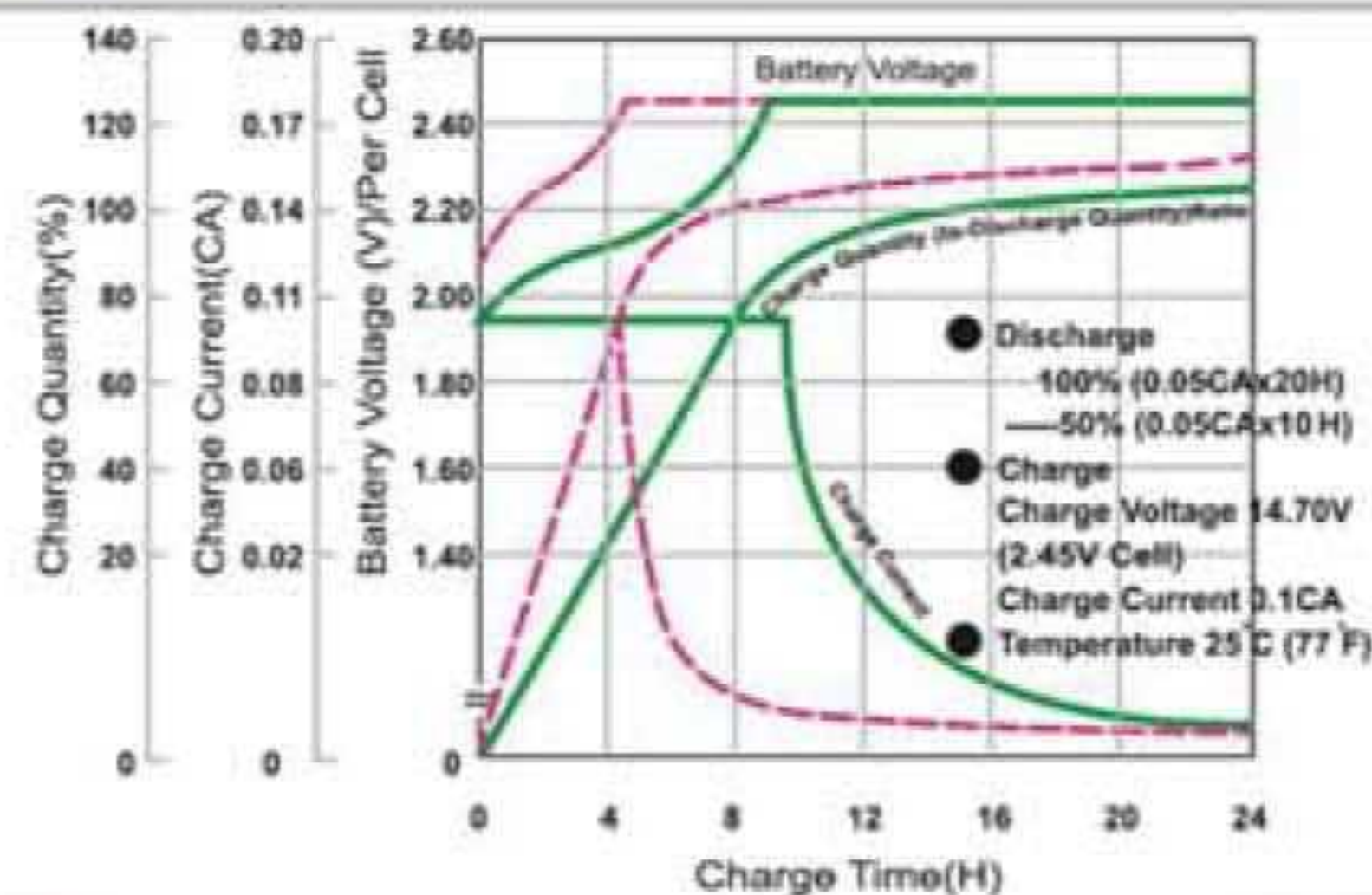
نمودار منحنی شارژ در حالت استفاده
