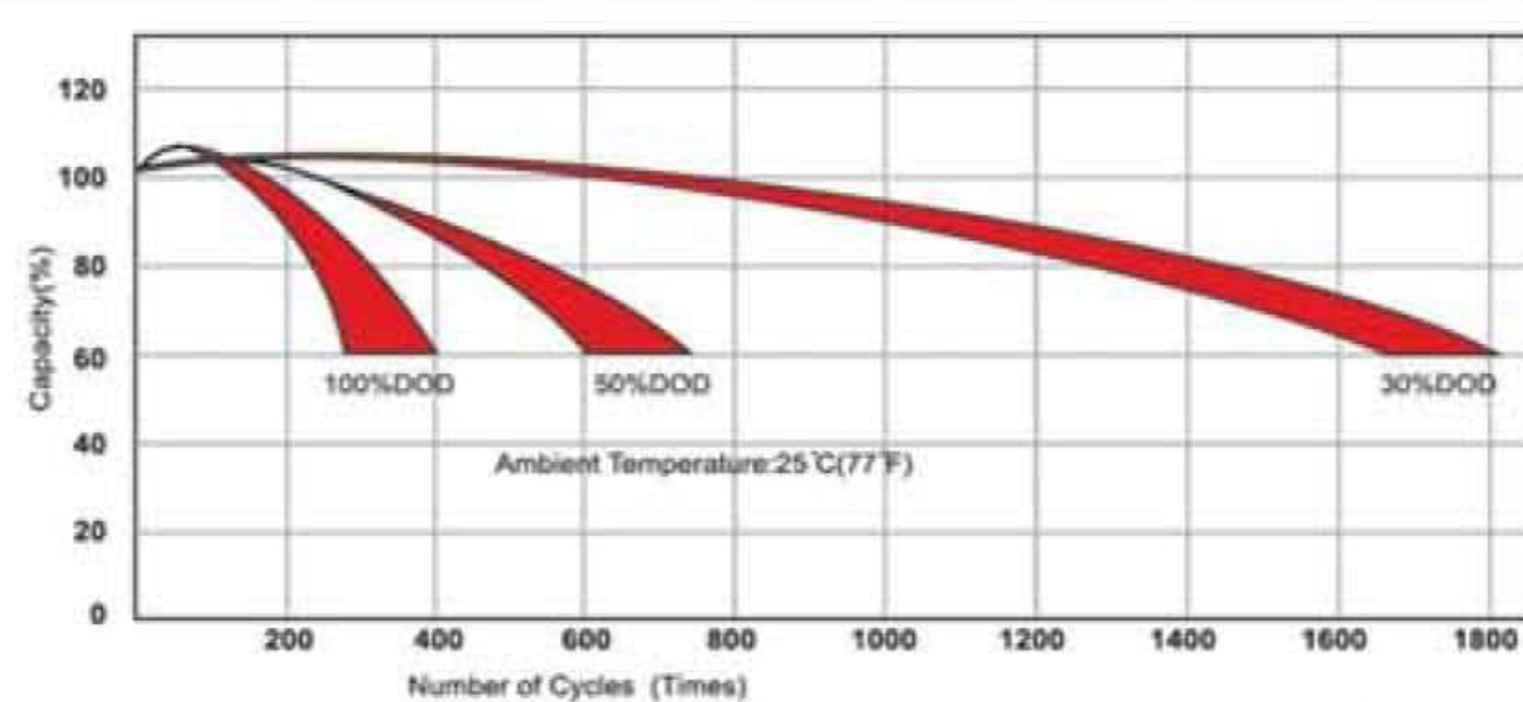
نمودار چرخه عمر نسبت به عمق دشارژ
