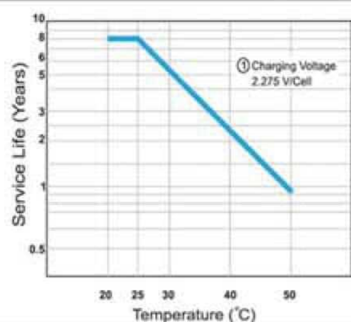
نمودار طول عمر در دمای متغیر
