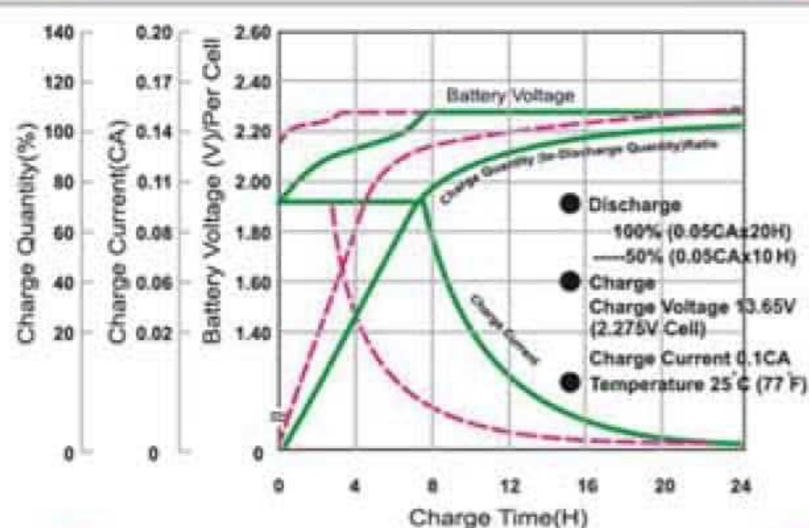
نمودار منحنی شارژ در حالت آماده بکار
