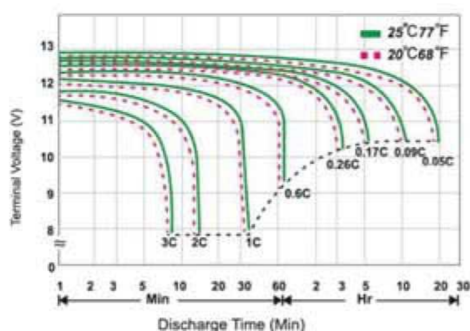
نمودار دشارژ
