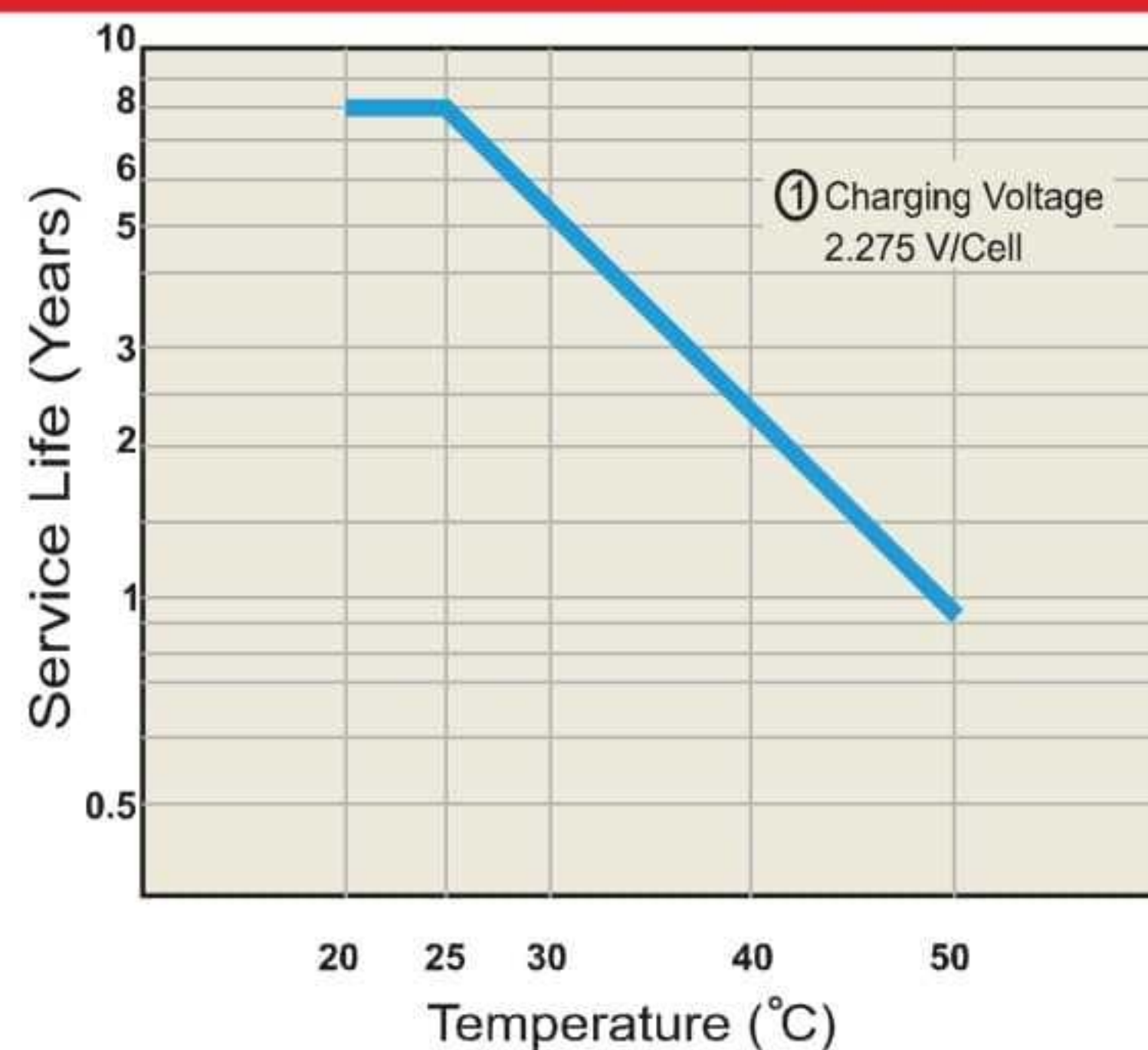
نمودار طول عمر در دمای متغیر
