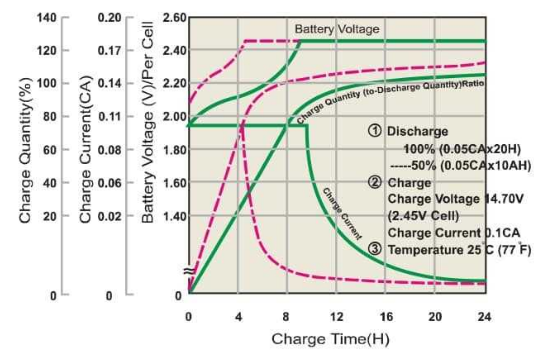
نمودار منحنی شارژ در حالت استفاده
