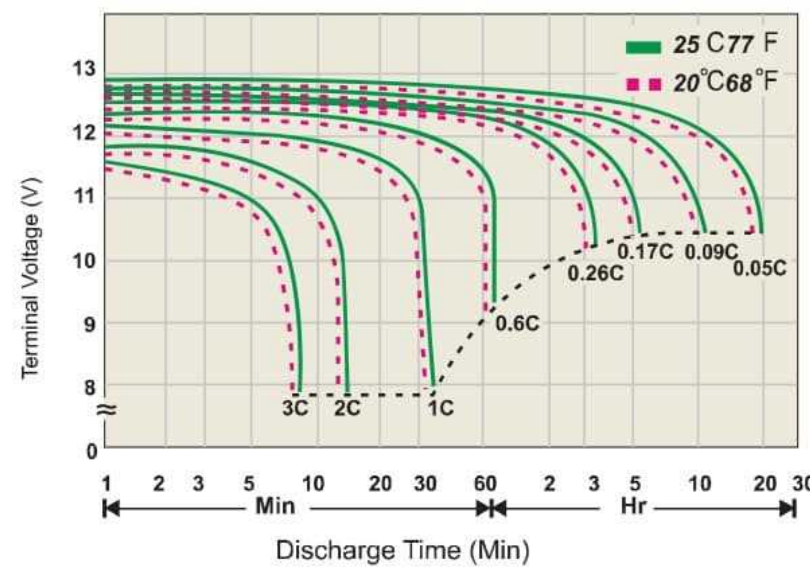
نمودار دشارژ
