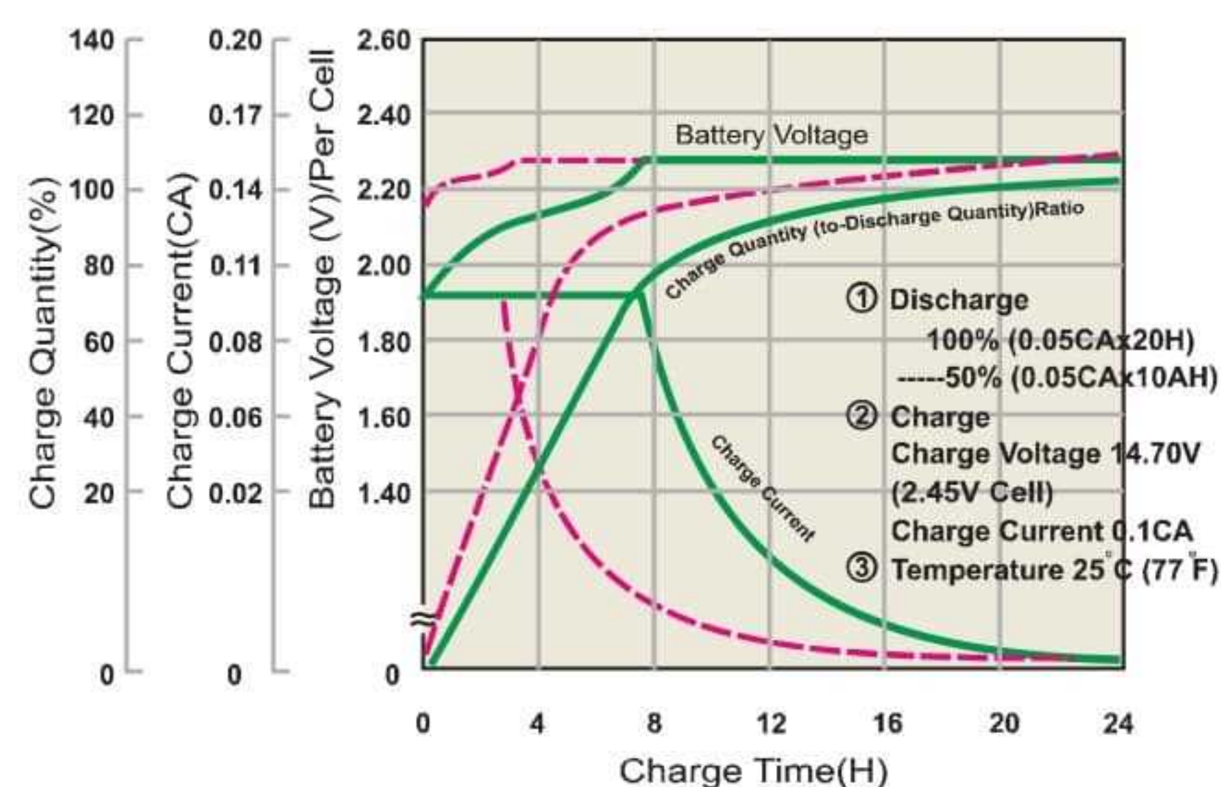
نمودار منحنی شارژ در حالت آماده به کار
