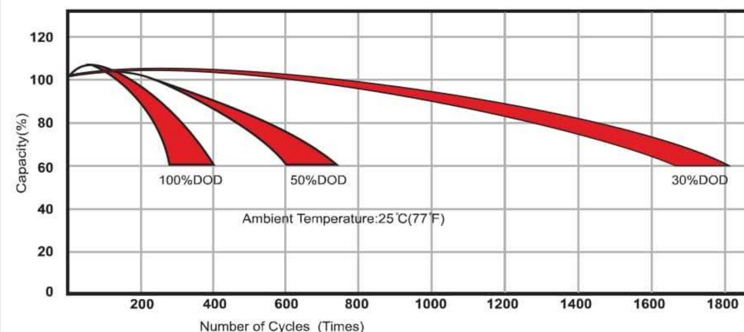
نمودار چرخه عمر نسبت به عمق دشارژ
