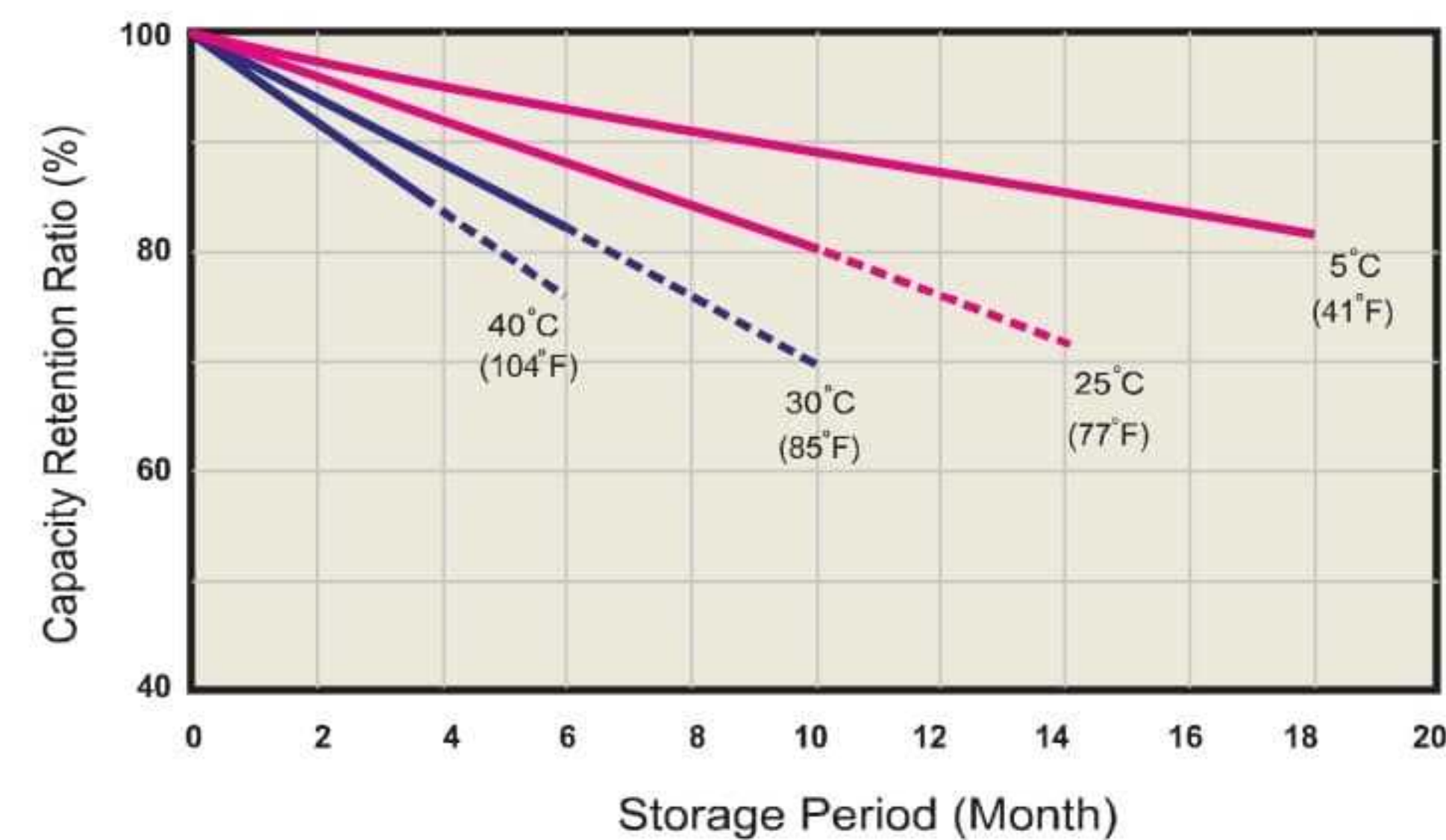
نمودار مشخصه حفظ ظرفیت
